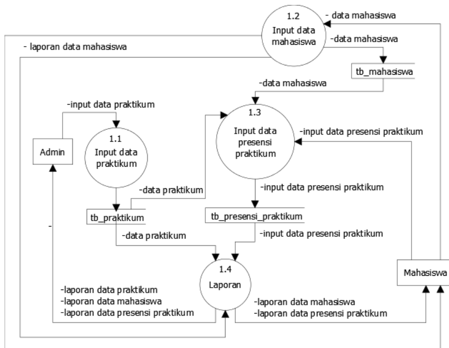
Gambar 4 DFD Level 1
